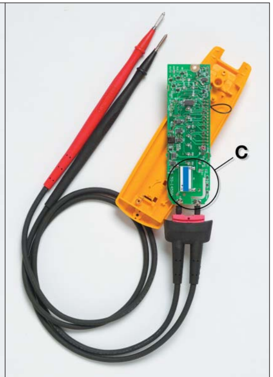
Figuur 2: Deze elektronische tester wordt beschermd door stroombegrenzende weerstanden (zie C), die ervoor zorgen dat de tester op voorspelbare wijze zal reageren wanneer deze aan elektrische impulsen wordt blootgesteld.
